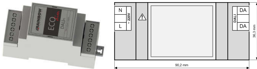
Рисунок 1. Общий вид и габаритные размеры.
